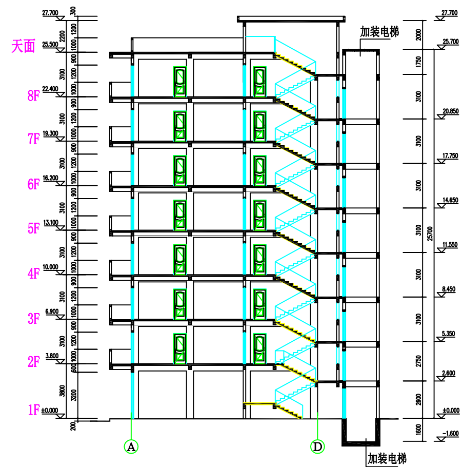
A-A剖面图
