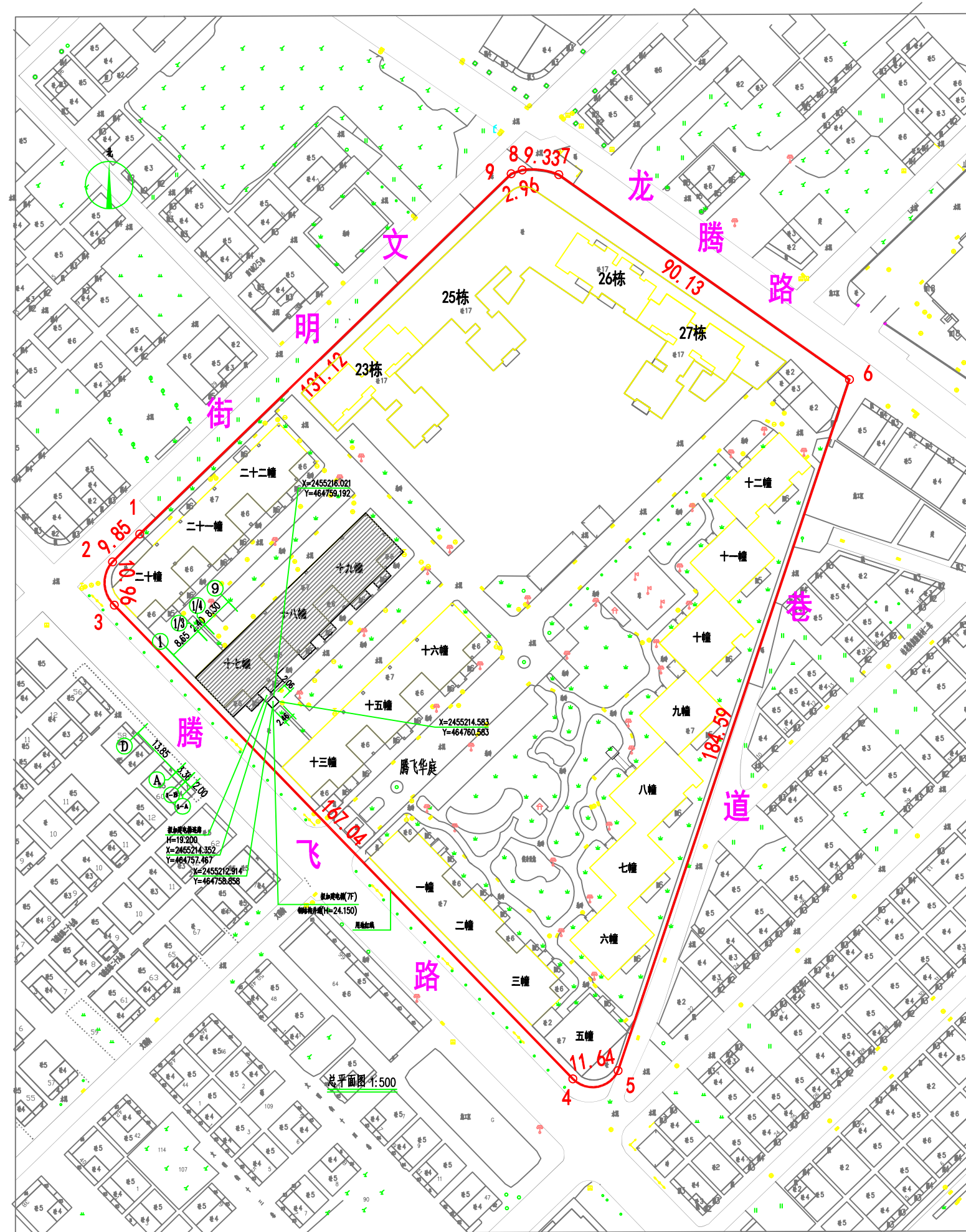
总平面图
