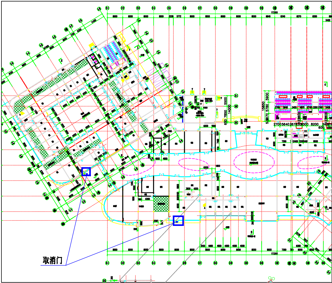
原方案东区服务楼一层建筑平面图
