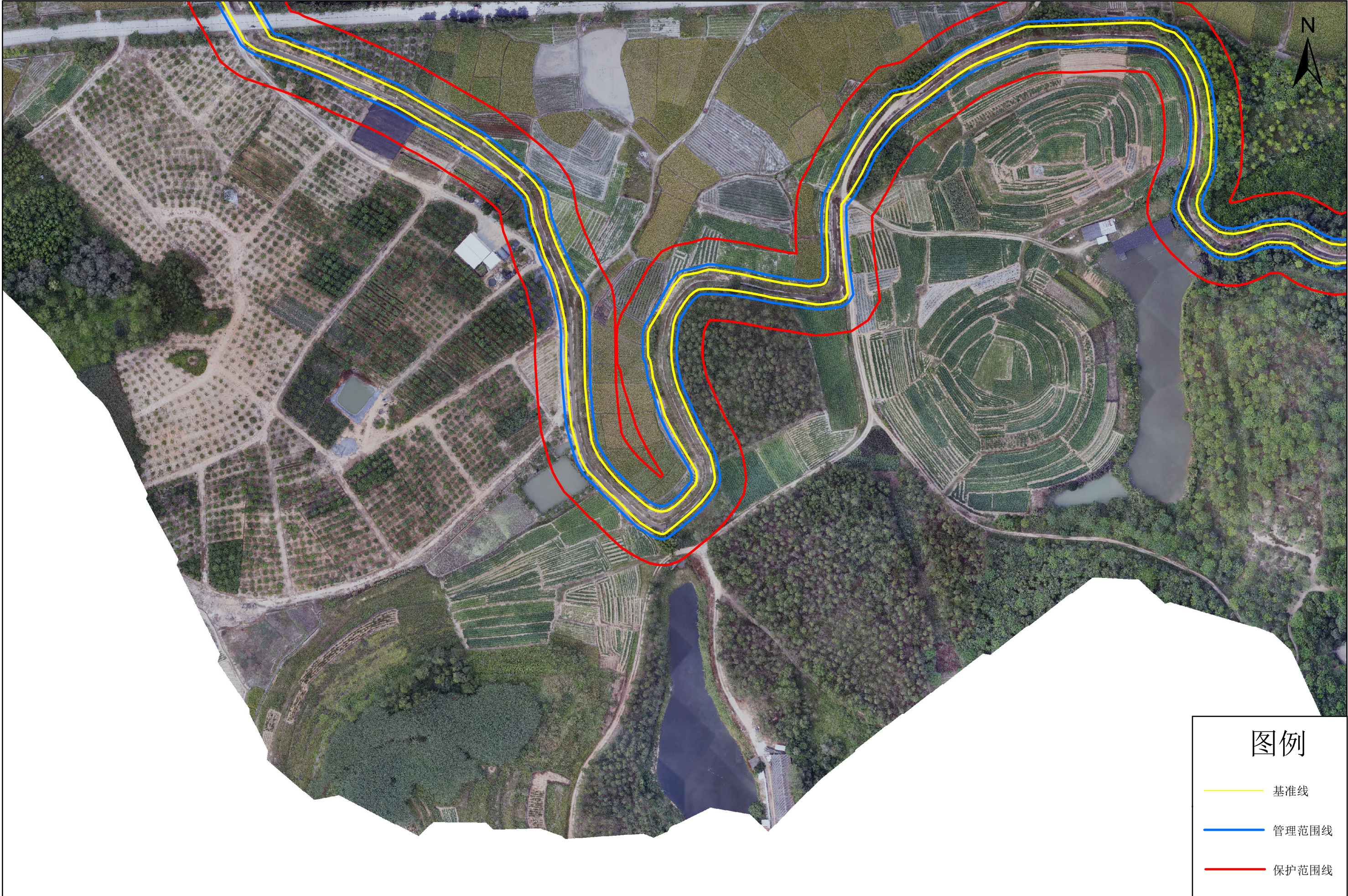
恩平市良西灌区管理与保护范围划定成果图 14 /32
