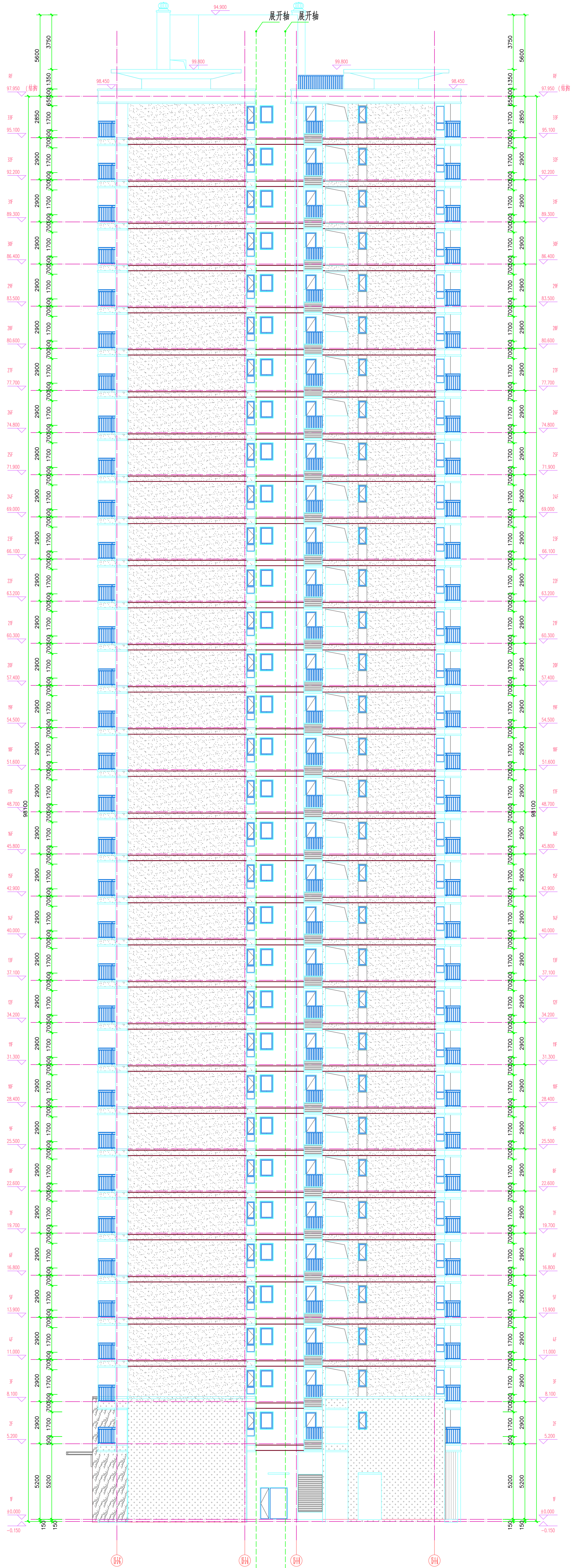
轴展开立面图 1:100
