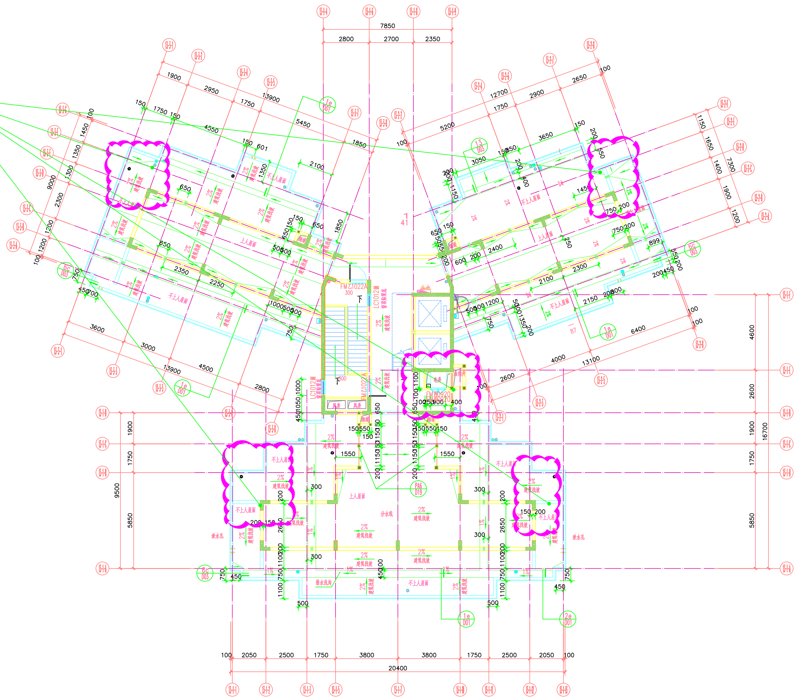
13#楼屋顶平面图 1:100
