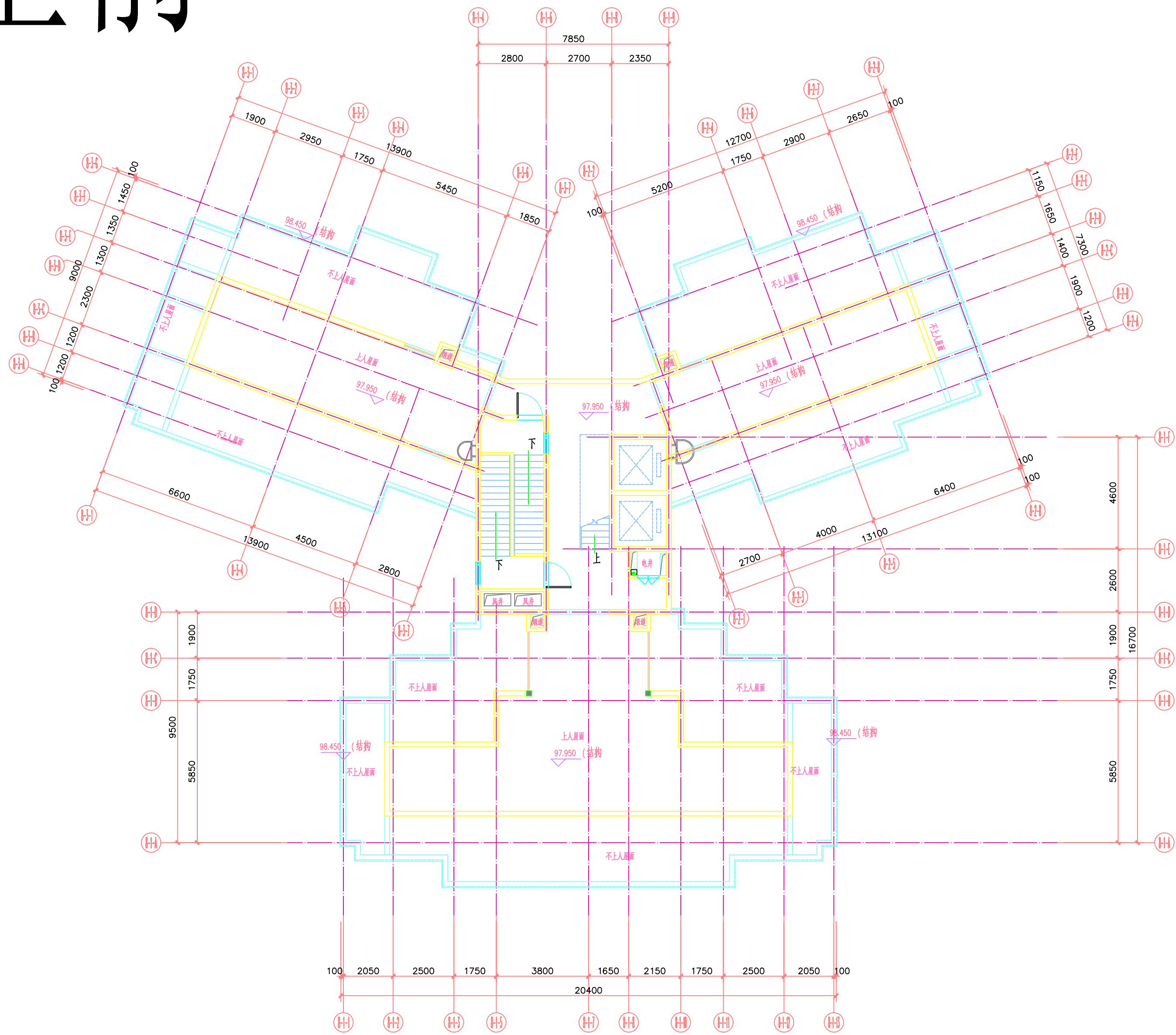
屋面层平面图 1:100
