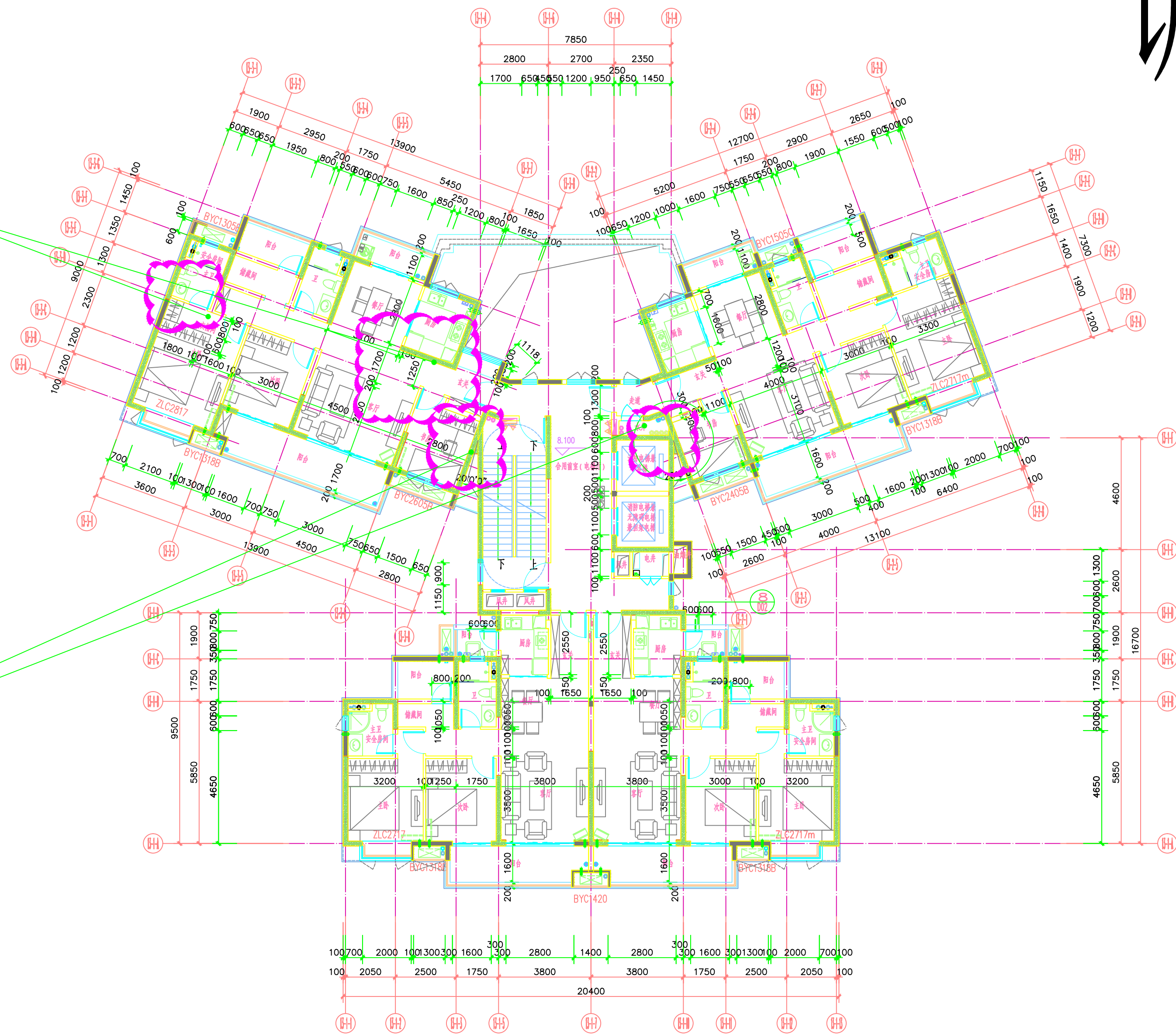
13#楼三层平面图 1:100
