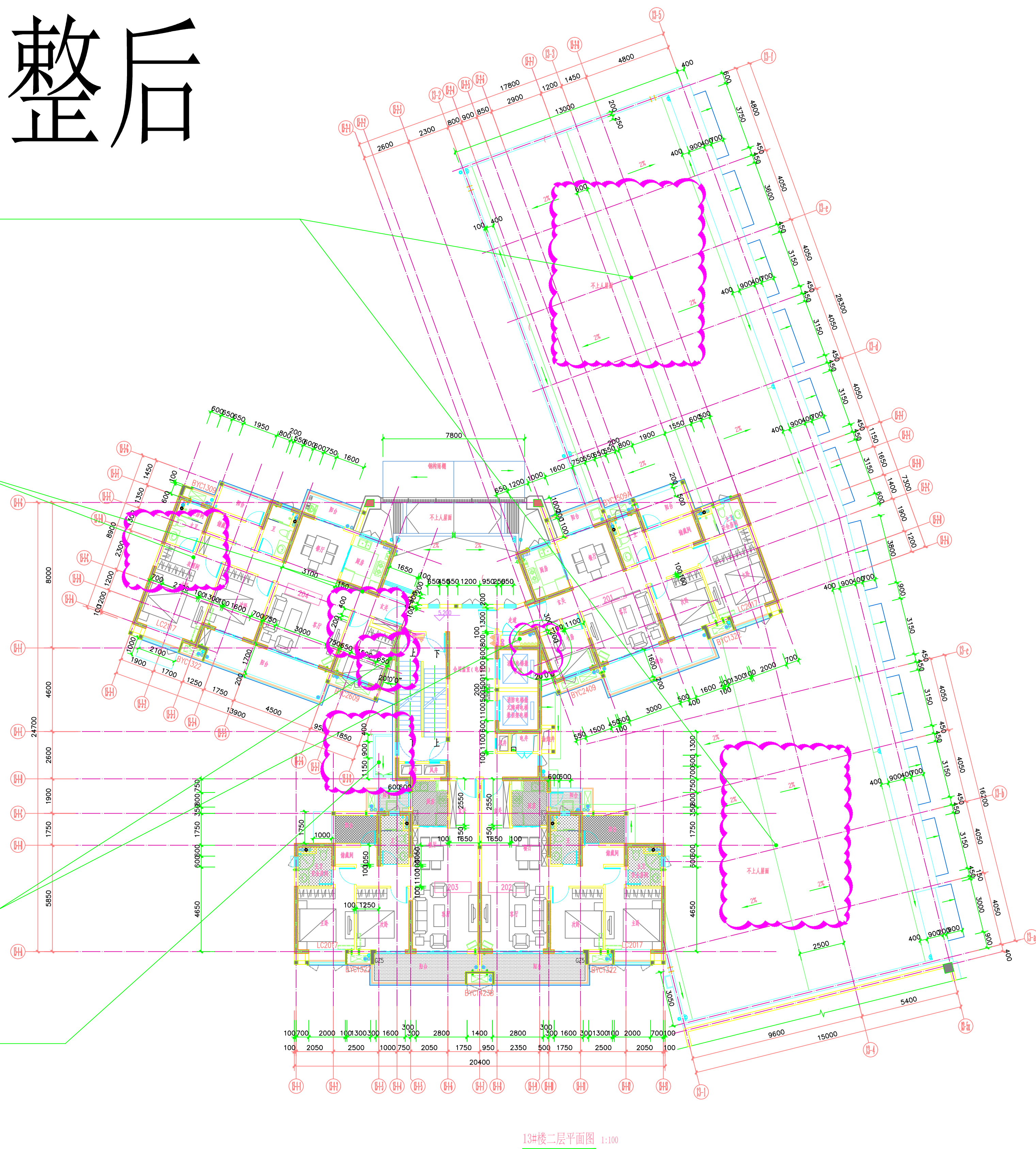
13#楼二层平面图 1:100
