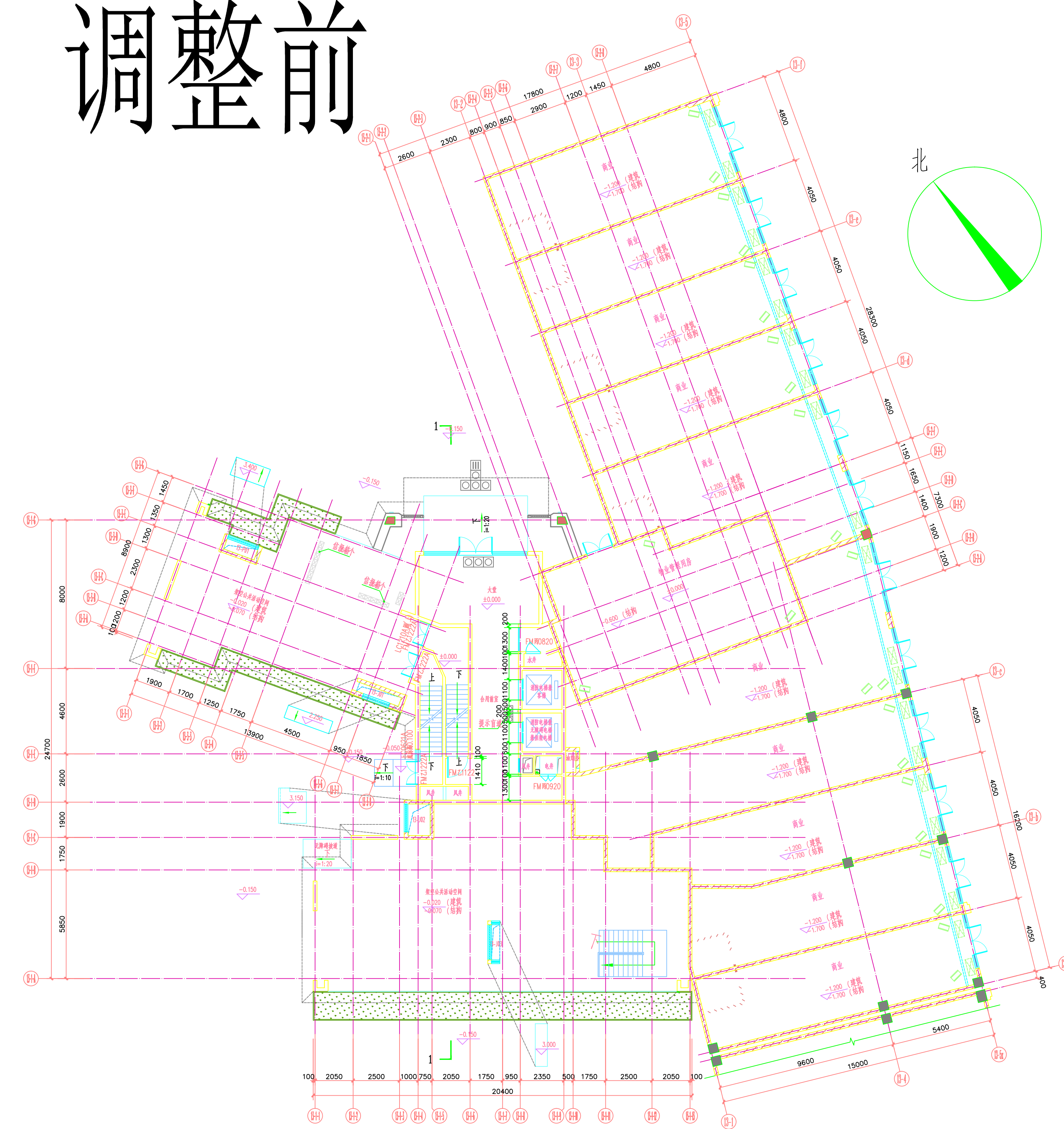
一层平面图 1:100
