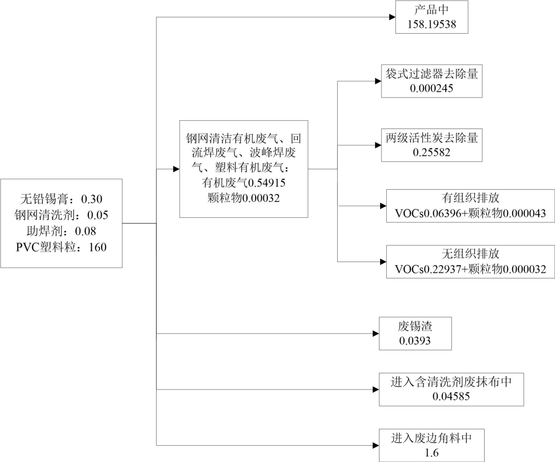
图 2-1 项目含 VOCs 物料平衡图 单位：t/a
