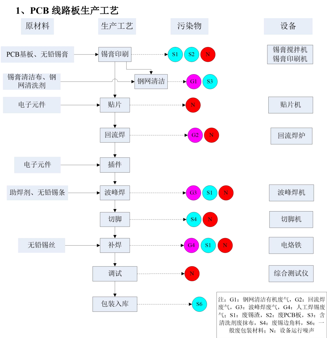
图 2-3 项目 PCB 线路板生产工艺流程及产污环节
