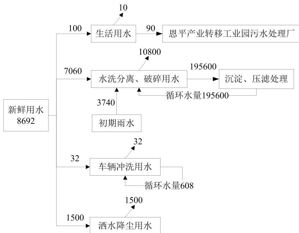
图 2-1 本项目水平衡图 单位：m³/a
