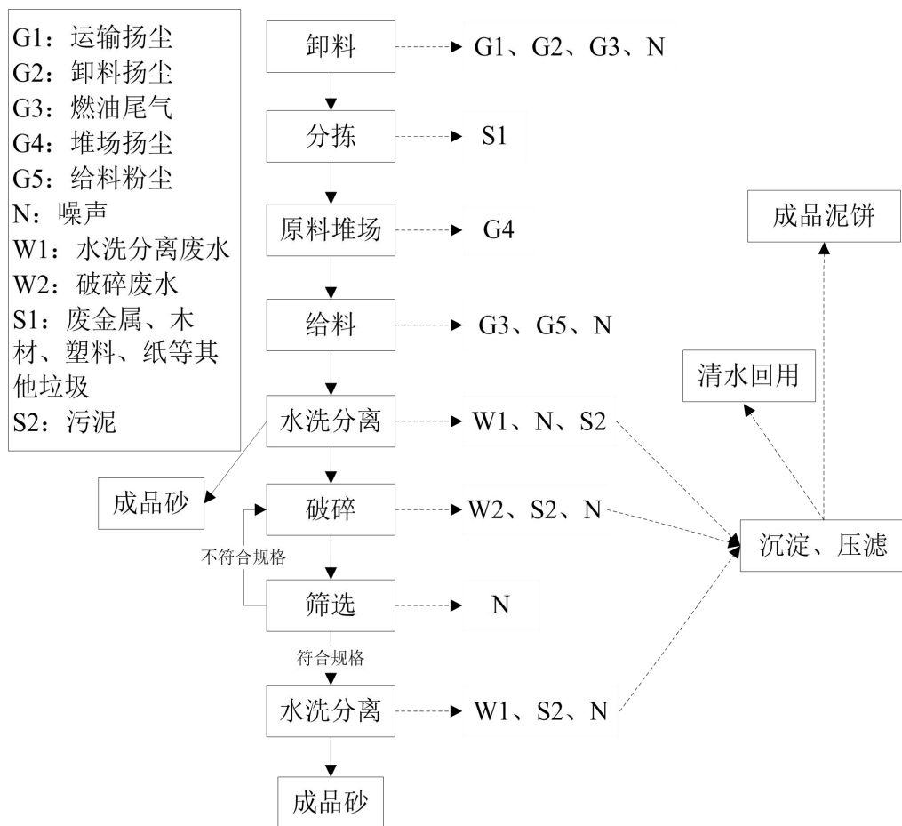
图 2-2 本项目生产工艺流程及产污环节图
